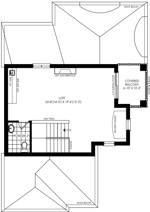
LOFT PLAN ELEV. 'D'
