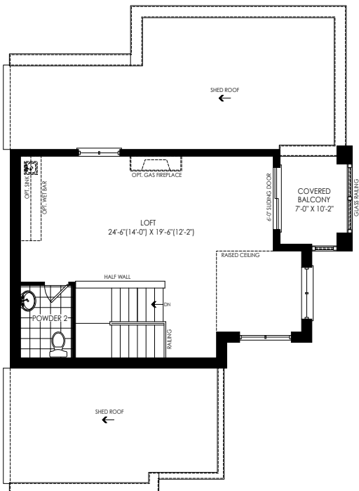
LOFT PLAN ELEV. 'A'
