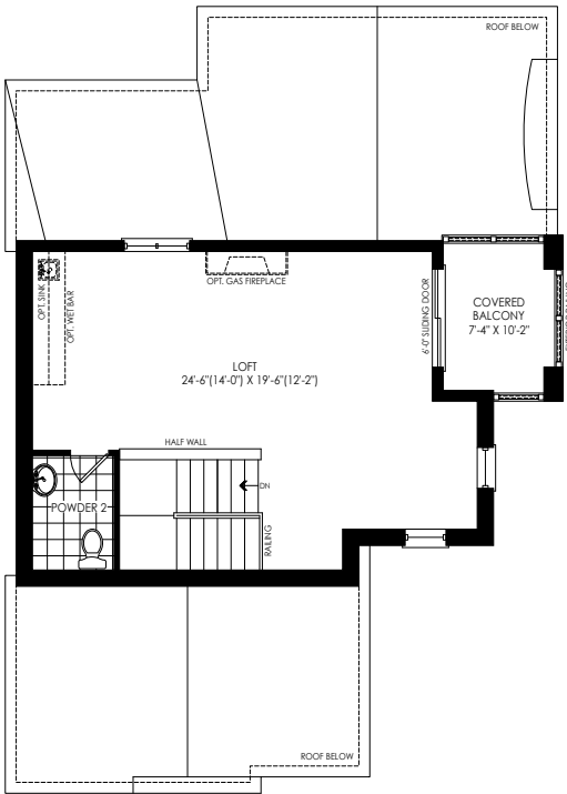
LOFT PLAN ELEV. 'B'
